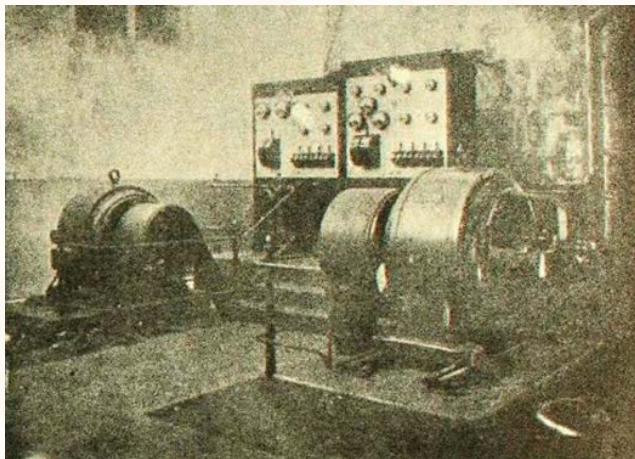
Máquina a vapor Sulzer Tandem. Revista Zig-Zag , diciembre de 1911.
